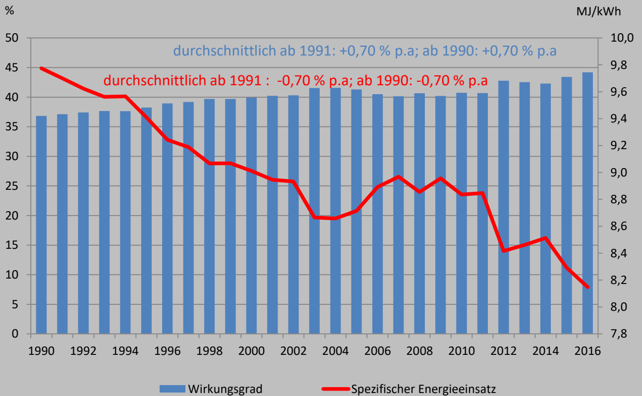
Wirkungsgrad und spezifischer Energieeinsatz der Stromerzeugung 1 - 1990 bis 2016
