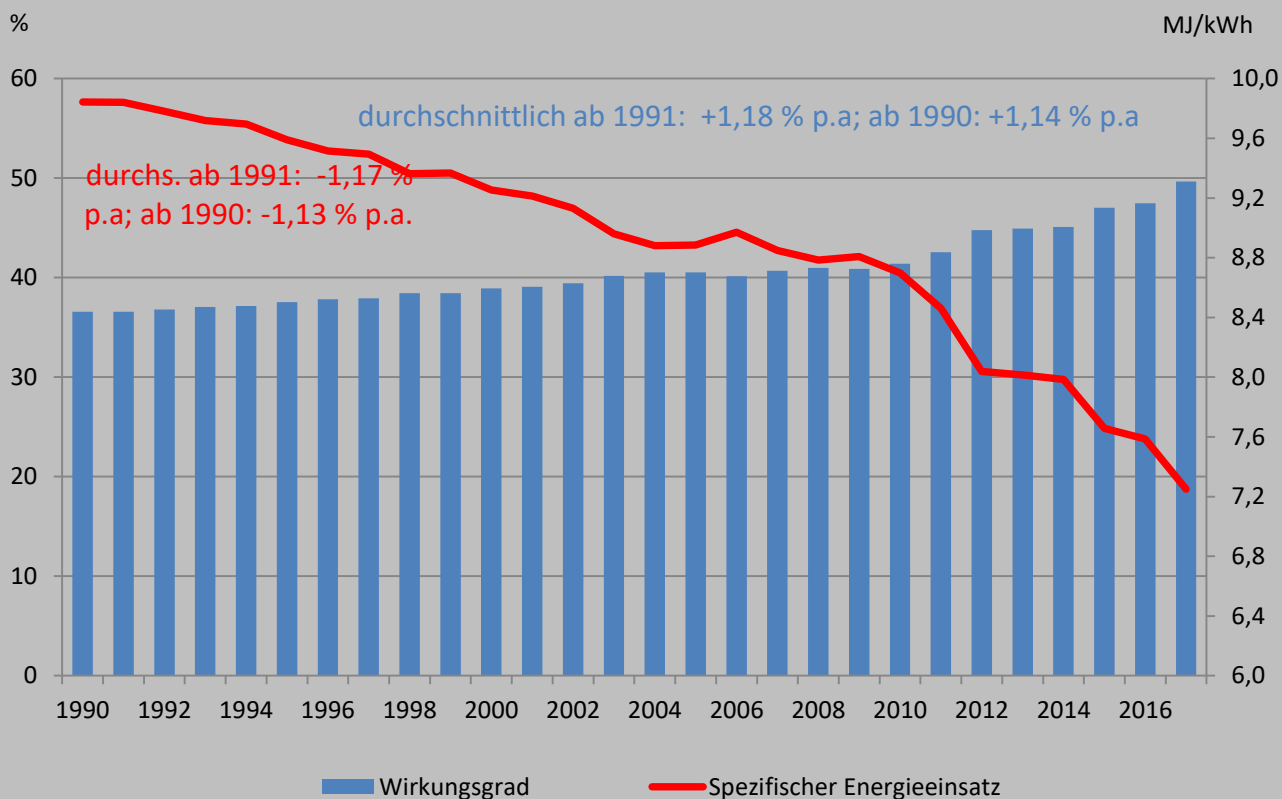
Wirkungsgrad und spezifischer Energieeinsatz der Stromerzeugung 1
